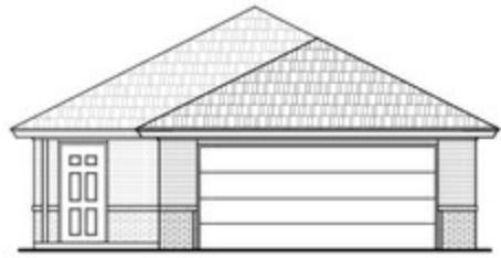
2 S1 ELEVATION A SCALE: 1/8" = 1'-0"
